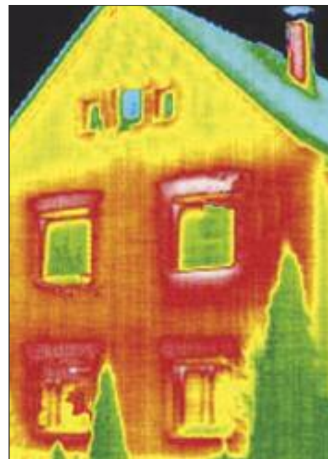
Abbildung zeigt eine Thermographieaufnahme
