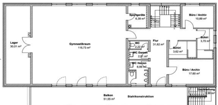
Obergeschoss: Büro für Fußballbetrieb und Vereinsführung. 2 Kabinen für Schiedsrichter inkl. Duschen, Mehrzweckraum inkl. Lager für Sportbetrieb und Veranstaltungen.
